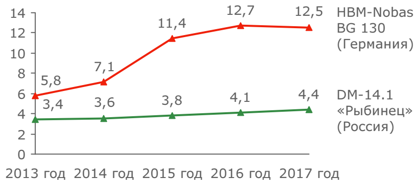
АВТОГРЕЙДЕРЫ, млн. руб.
